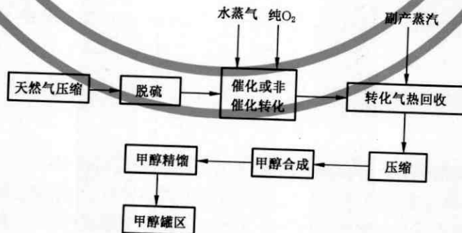
图 A.5 以天然气为原料生产甲醇的典型生产工艺流程
